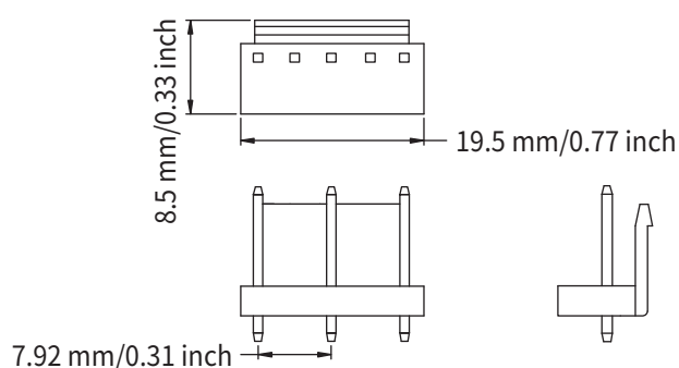
CN1
